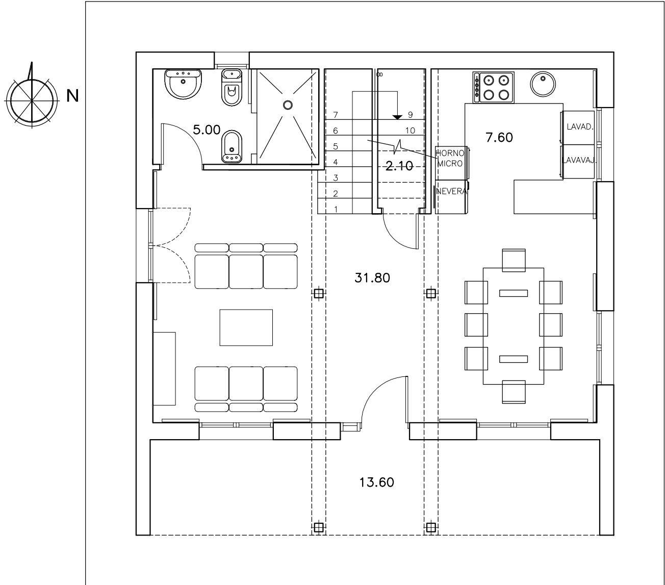
PLANTA BAJA
