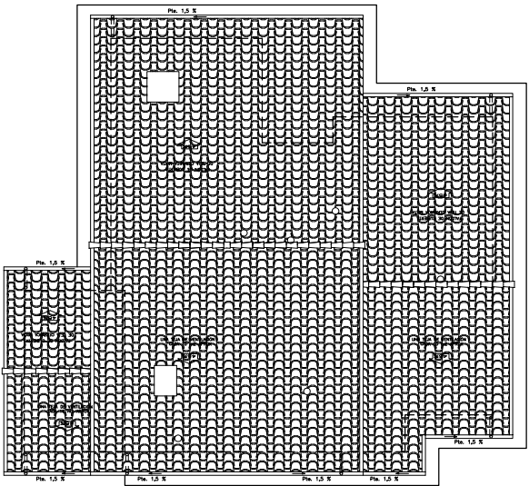
PLANTA CUBIERTA E: 1/100
